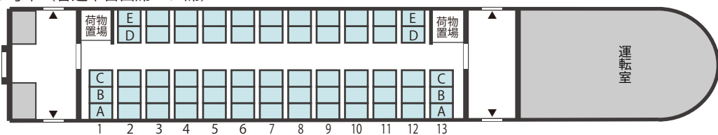
6号車 (普通車自由席 61席)
